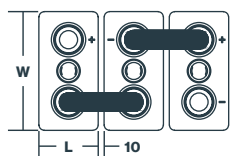
2 OPzS-ET200 to 7 OPzS-ET700
