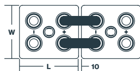
8 OPzS-ET800 to 13 OPzS-ET1625
